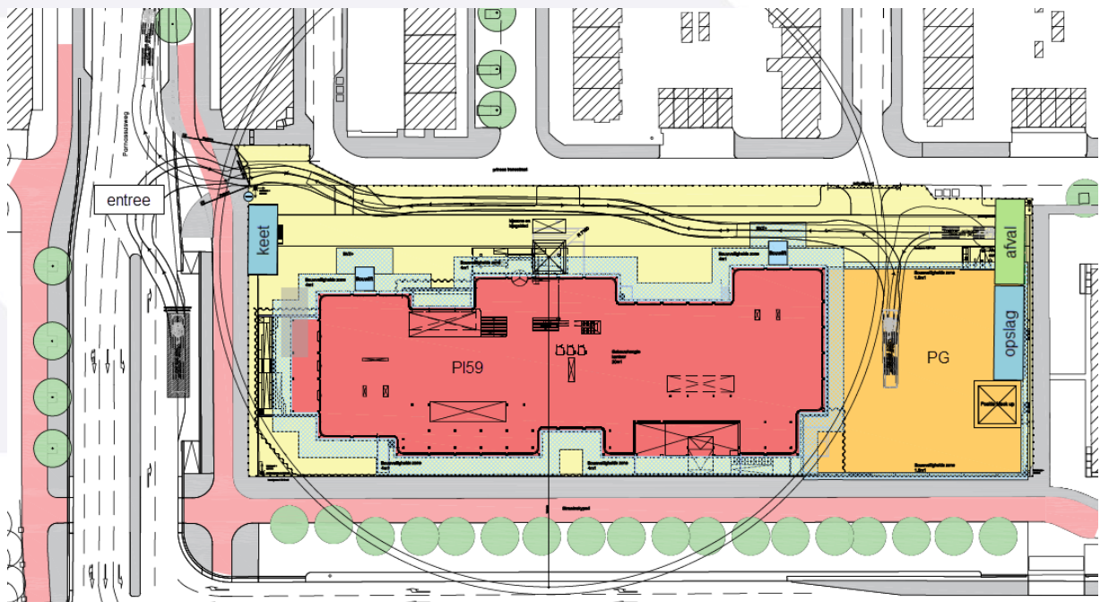
afbeelding 2; bouwplaatsinrichting
